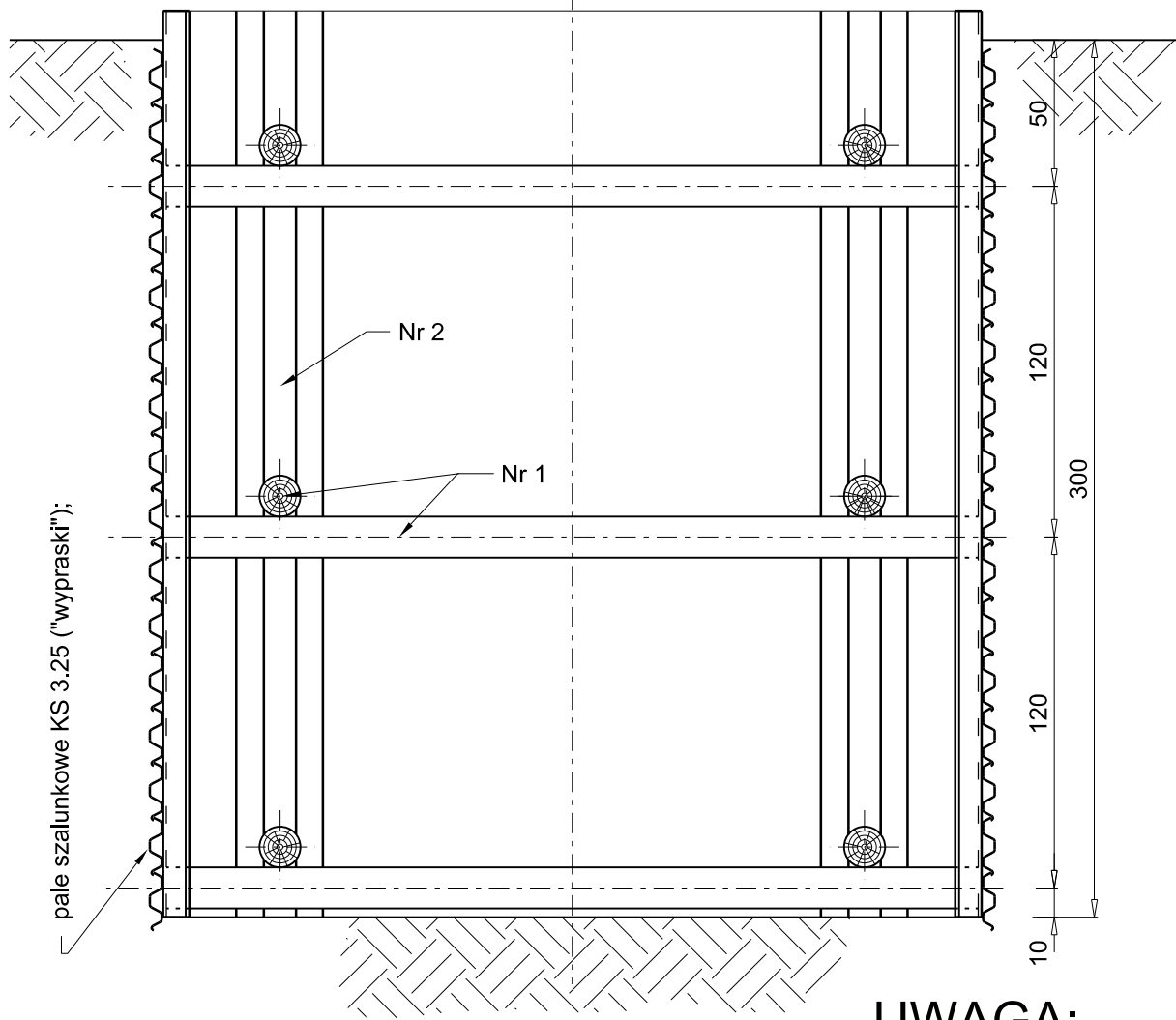
PRZEKRÓJ PIONOWY
