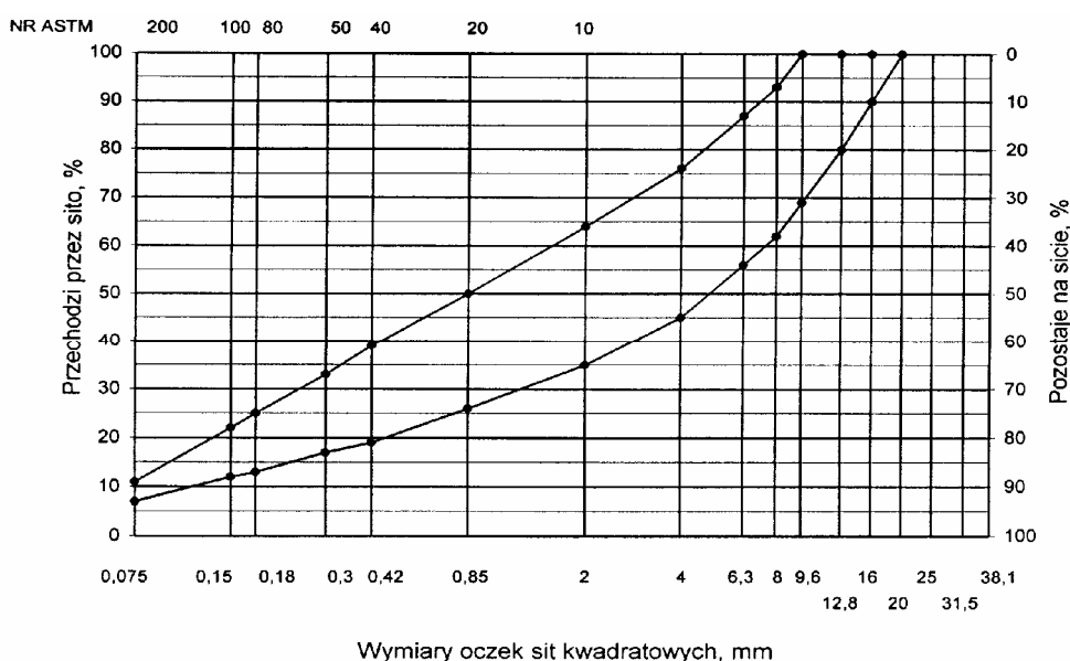
Rys. 1. Krzywe graniczne uziarnienia mieszanki mineralnej BA od 0 do 16mm, od 0 do 12,8 mm do warstwy ścieralnej i wiążącej nawierzchni drogi o obciążeniu ruchem KR1 lub KR2
